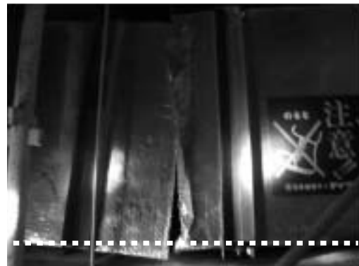
天井裏空調ダクトのずれ（点線が通常 の位置）
